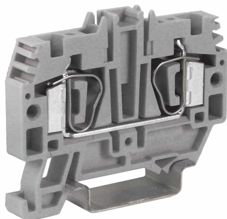
Morsetto a molla 4mm 2 , 1-piano, colore blu
