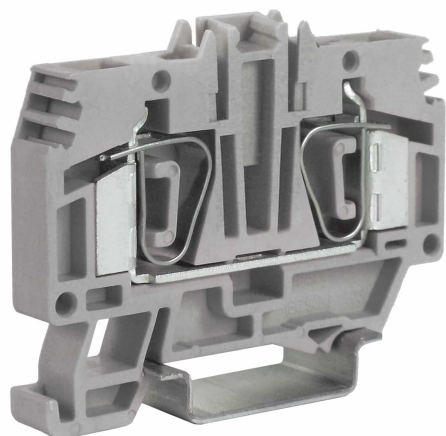
Morsetto a molla 6mm 2 , 1-piano, colore grigio
